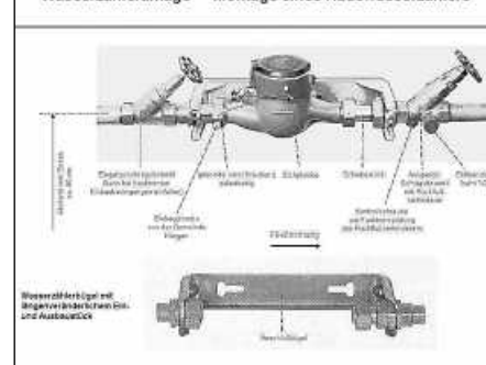
Wasserzähleranlage - Montage eines Hauswasserzählers
